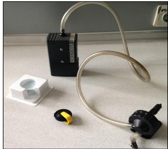
Resim 3.2 Kişisel hava örnekleme pompası, siklon başlık, PVC filtre ve filtre kaseti
