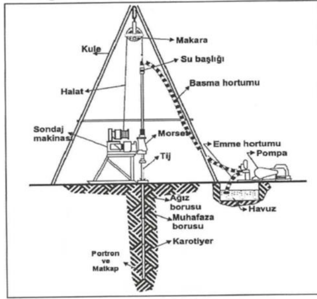
Resim 2.2. Sondaj makinesinin ana üniteleri [8]
