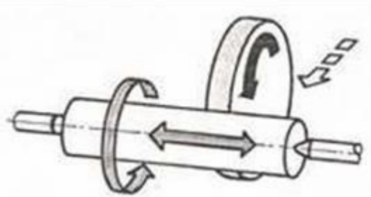
Şekil 2.4. Taşlama işlemi [14]
