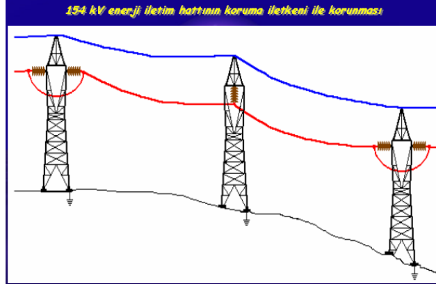
Şekil 16: Koruma İletkeni
