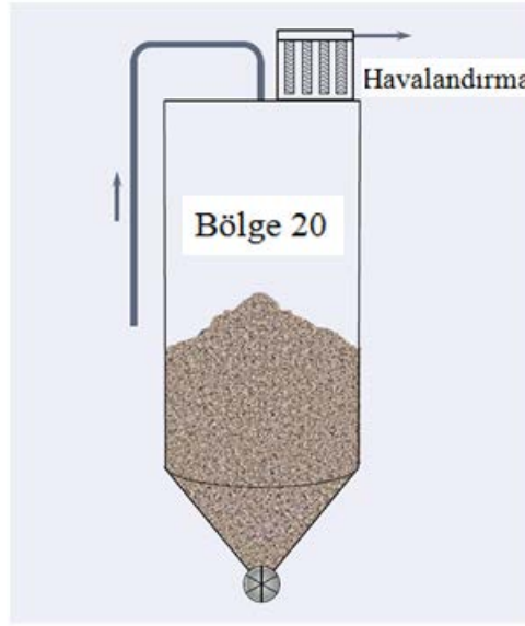
Şekil 5. Patlayıcı toz ihtiva eden siklonda tehlikeli bölge sınıflandırması
