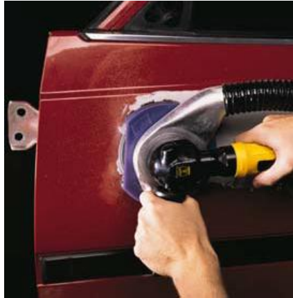
Şekil 8. El aletlerine montajlı emiş sistemi [11]
