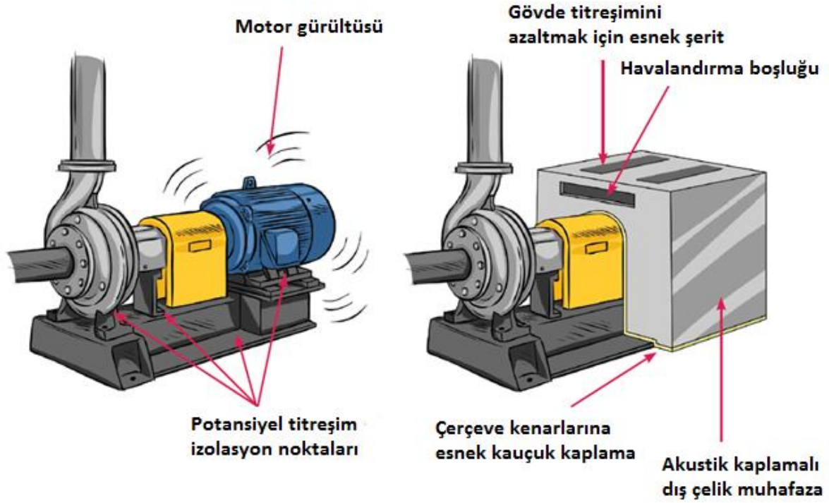
Şekil 2.23. Muhafazasız ve muhafazalı pompa motoru
