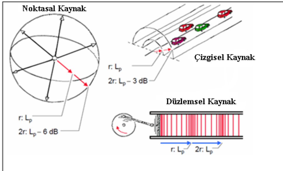
Şekil 2.11. Nokta, çizgisel ve düzlemsel ses kaynakları [15]
