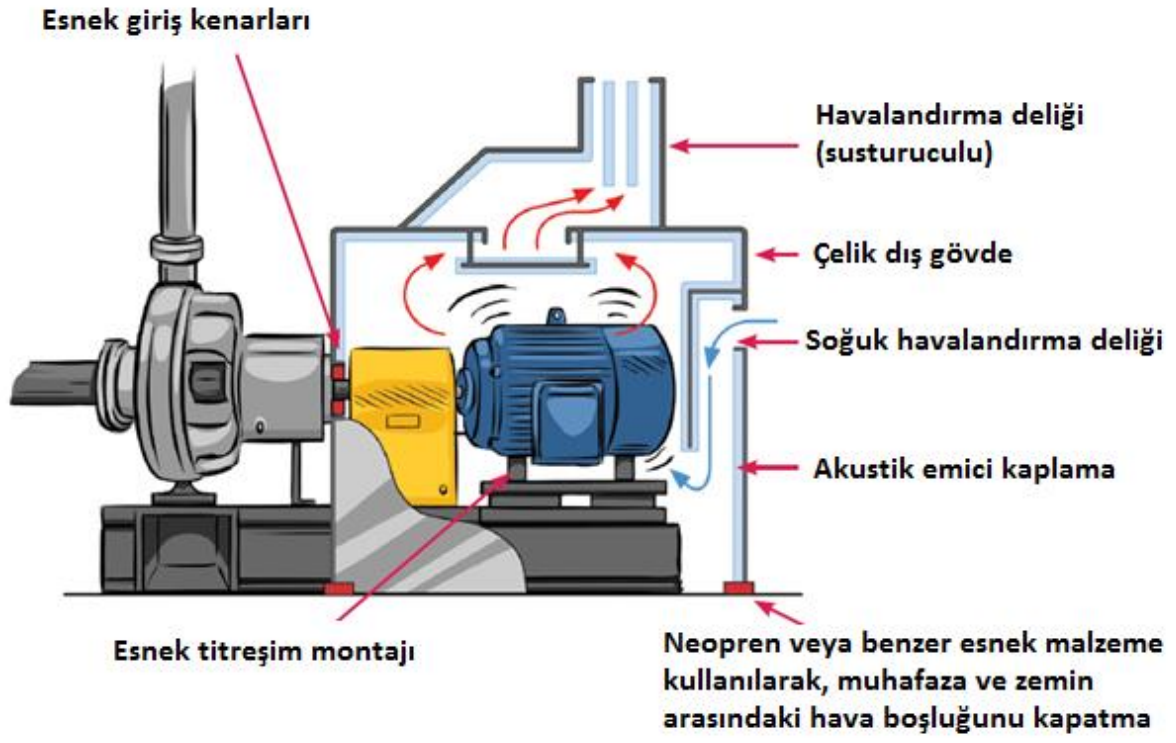
Şekil 5.12. Muhafazalı pompa motoru kesiti
