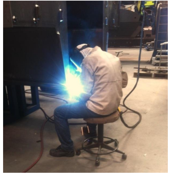
Resim 3.15. MIG-MAG kaynağı
