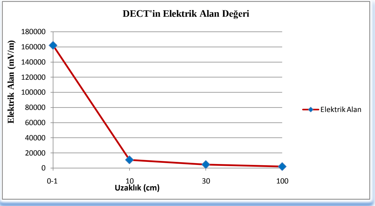
Resim 17. Uzaklığa Bağlı Olarak DECT İçin Elektrik Alan Değişimi
