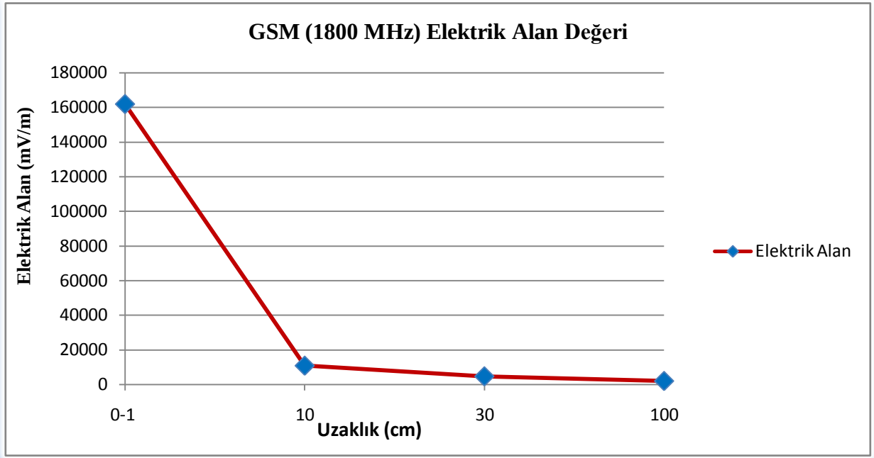
Resim 24. Uzaklığa bağlı olarak 1800 MHz için elektrik alan değişimi
