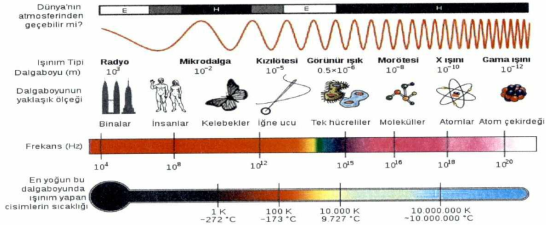
Resim 7. Elektromanyetik spektrumu
