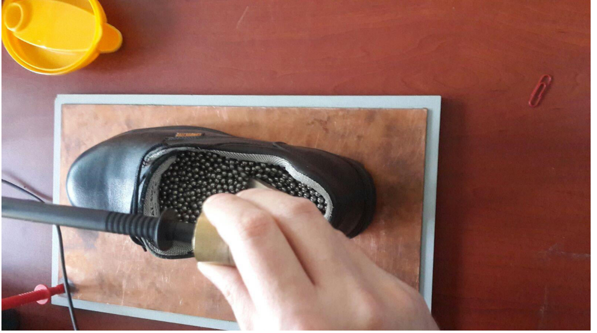
Resim 3.8.Cihaz uçlarının konumlandırılması
