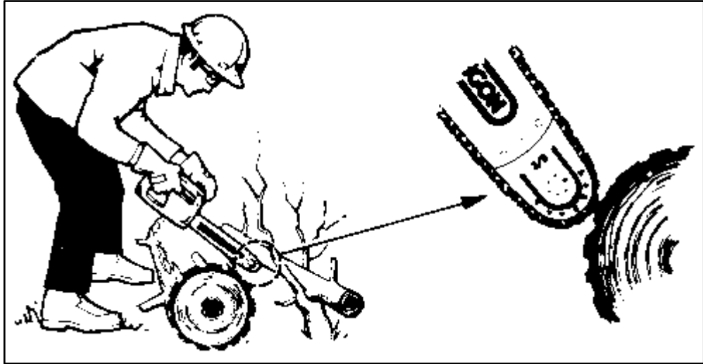
Şekil 2.1. Geri tepme [9]
