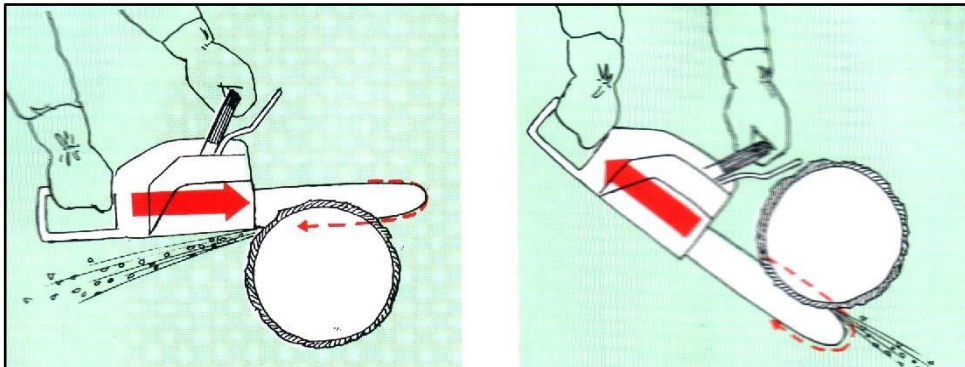
Şekil 2.12. Motorlu testere levhasının alt ve üst tarafıyla kesiş [8]
