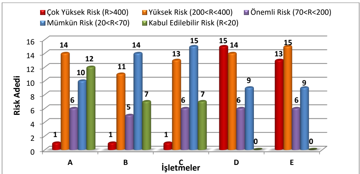
Şekil 4.26. Genel işyeri bölümlerinde tespit edilen risklerin risk düzeylerine göre dağılımı
